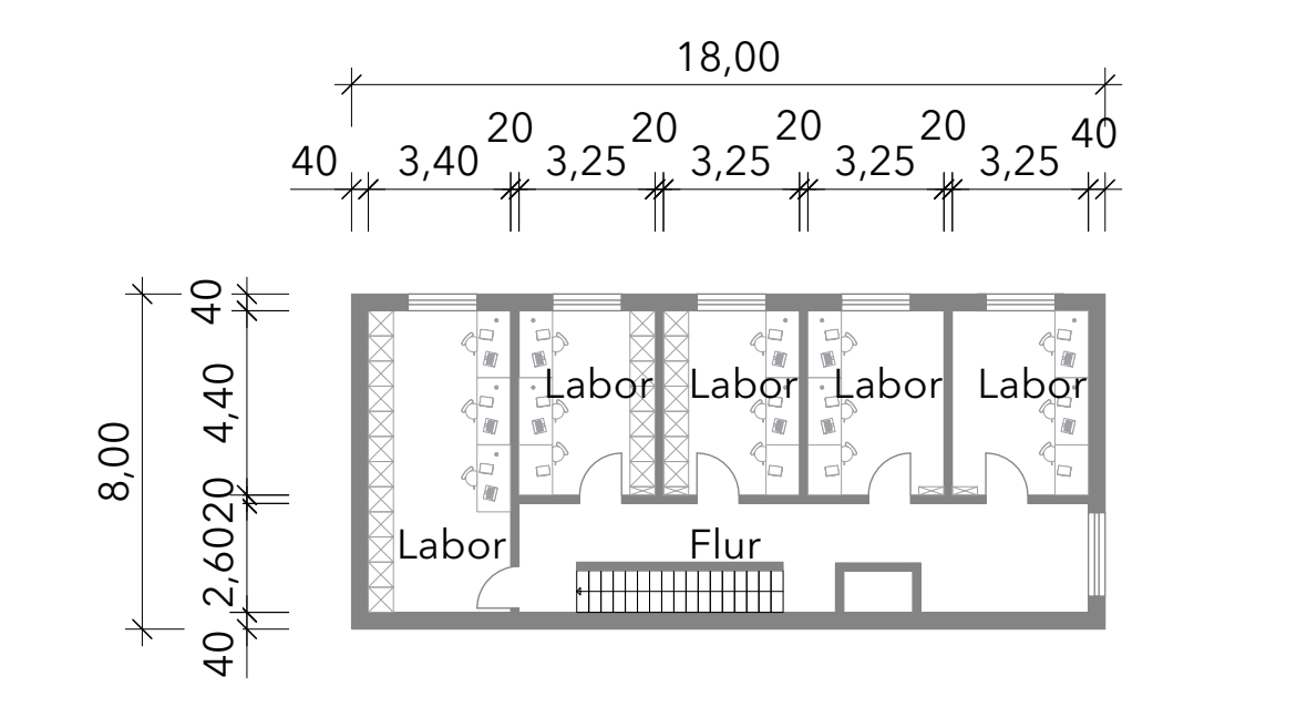
GRUNDRISS OBERGESCHOSS BÜROGEBÄUDE M 1:1.200
