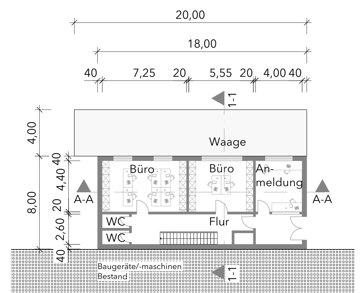
GRUNDRISS ERDGESCHOSS BÜROGEBÄUDE M 1:1.200
