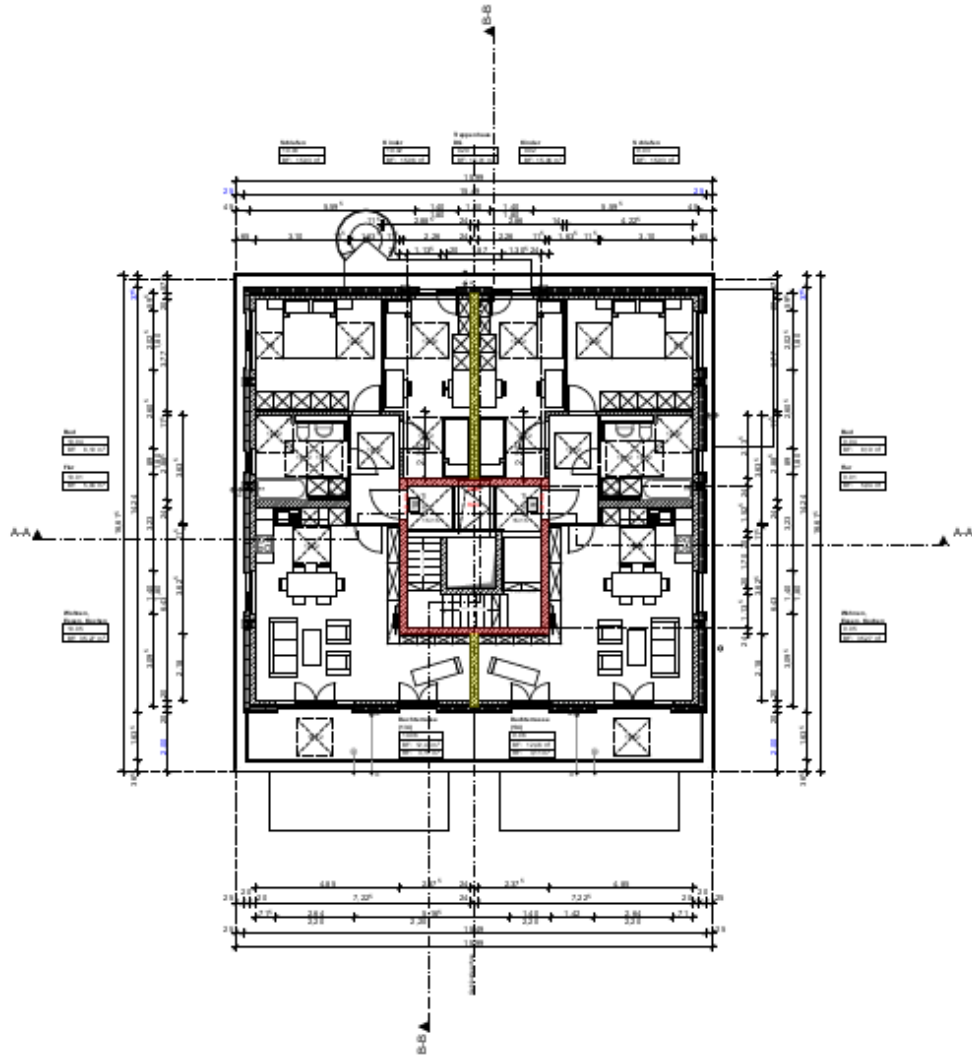
GRUNDRISS DACHGESCHOSS
